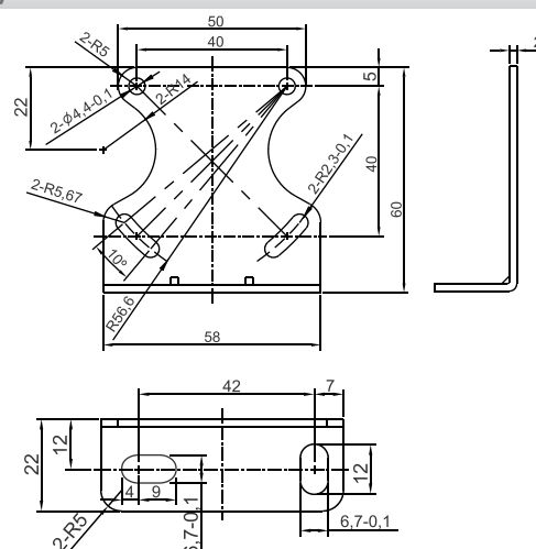
Suporte de montagem / Mounting suport
