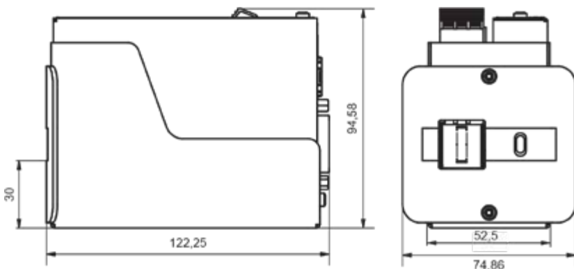
Desenho técnico com dimensões
